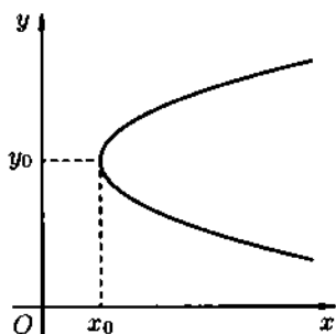
Рис. 43. (y - y_0)^2 = 2p(x - x_0)
